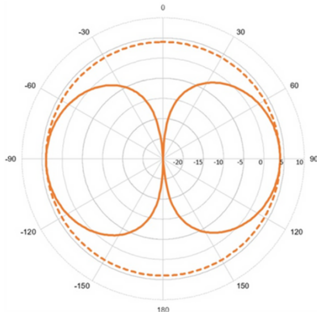
DT-11 Yayılım Paterni 150-170 MHz
