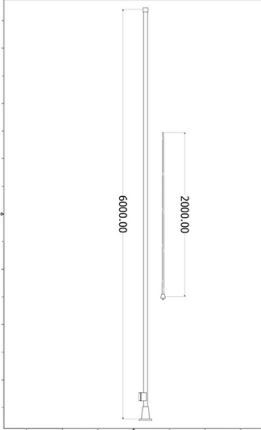
RESİM 1: Anten Ölçüleri
