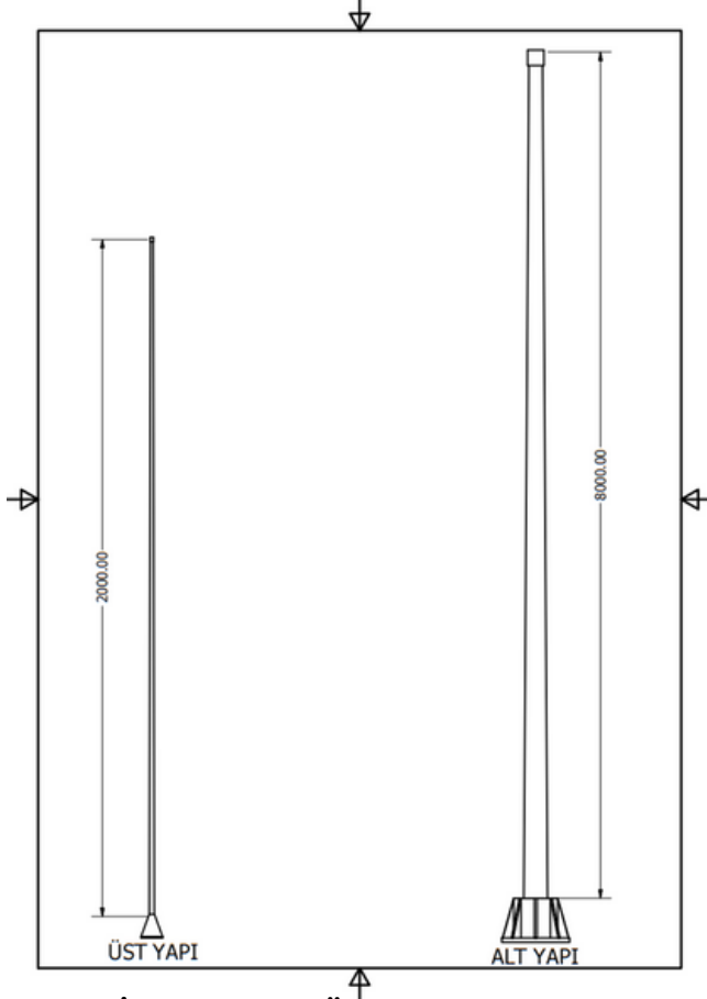
RESİM 1: Anten Ölçüleri
