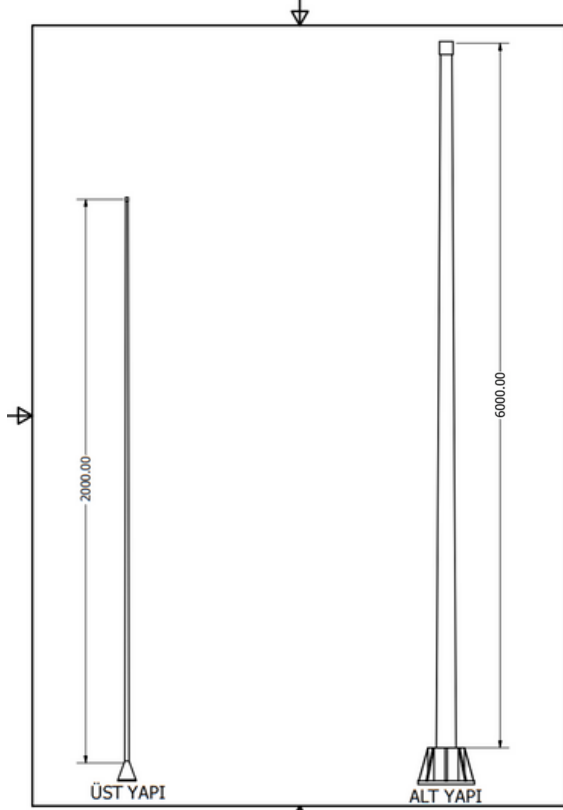
RESİM 1: Anten Ölçüleri
